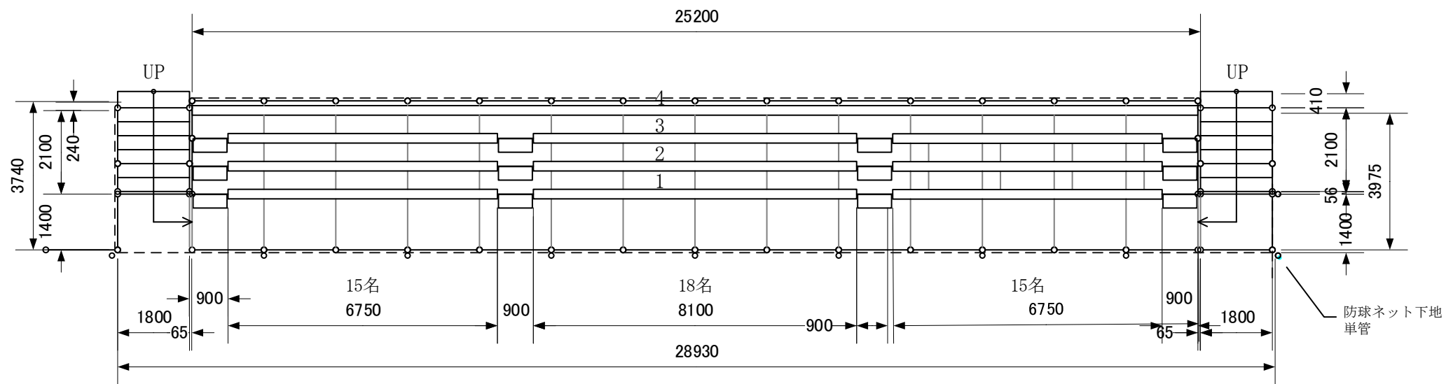
スタンド平面図 S=1/150 収容人員：200名×4基 = 800名(座席当たり45cm/名試算)
