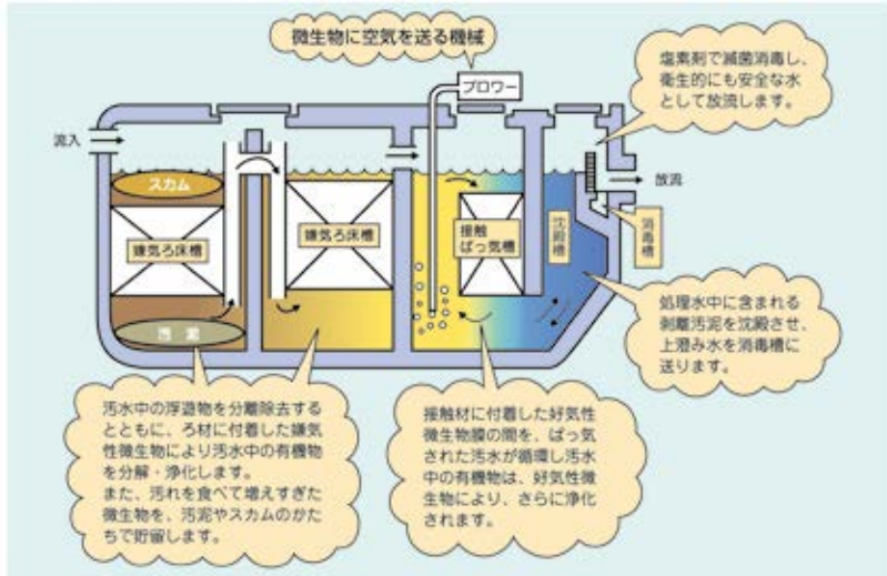
合併処理浄化槽の仕組み～きれいな水ができるまで～
