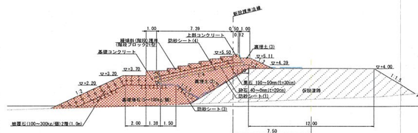
施工断面図
