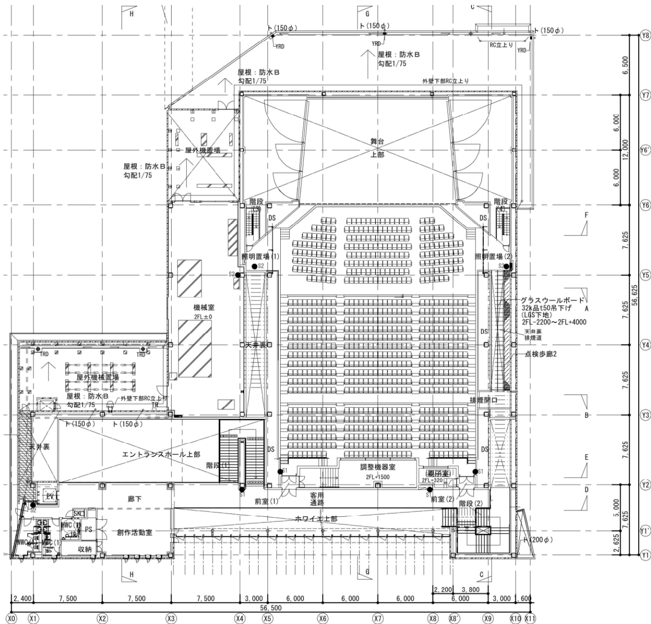
2階平面図
